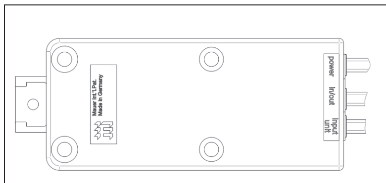
Abbildung 3: Schlossgehäuse
