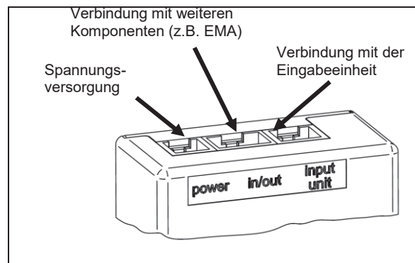
Abbildung 4: Anschlüsse am Schlossgehäuse
